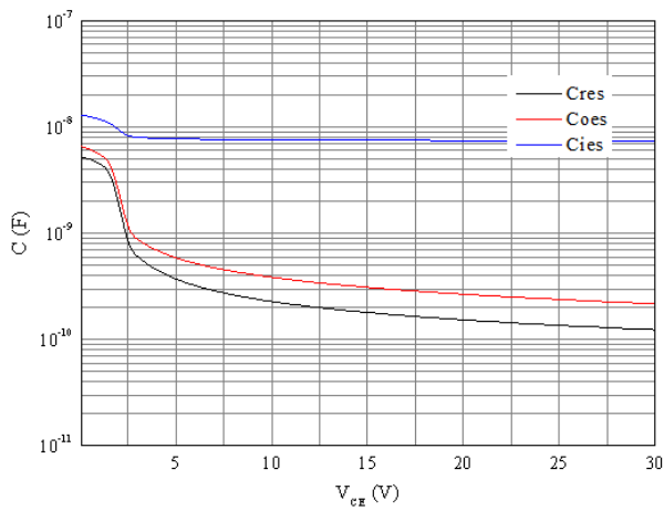
图 9. 电容特性
