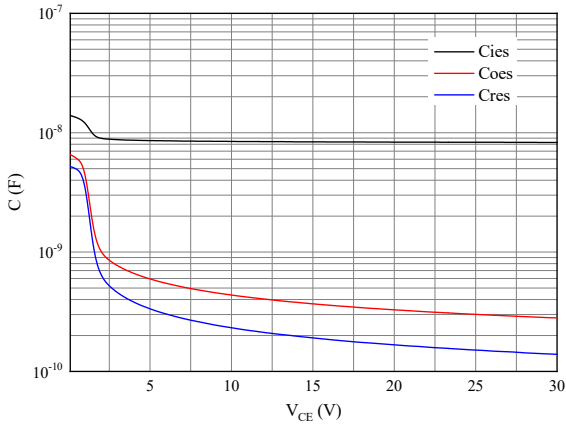
图 9. 电容特性
