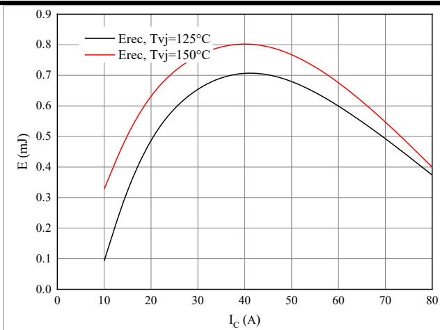
图 7. 开关损耗 二极管
