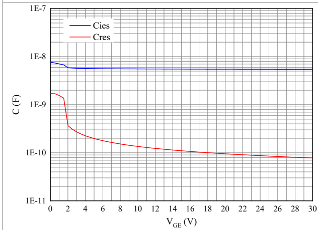
图 9. 电容特性
